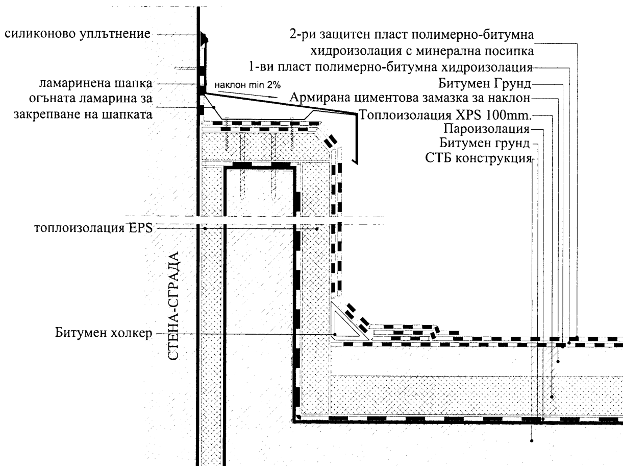
ОФОРМЯНЕ НА ДЕТАЙЛ ПРИ ВРЪЗКА СТЕНИ-ПОКРИВ
