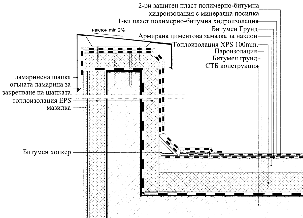
ОФОРМЯНЕ НА ДЕТАЙЛ ПРИ ВРЪЗКА БОРД-ПОКРИВ
